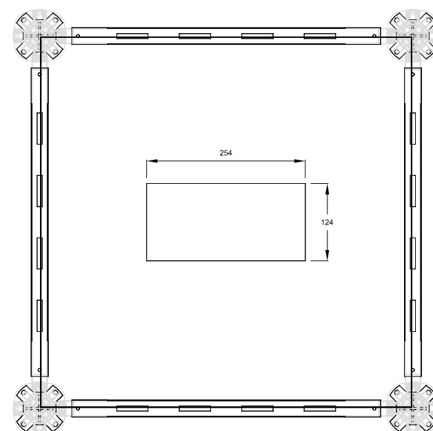
Dimensões de abertura no pavimento técnico sobreelevado Dimensions of opening in the raised technical floor
