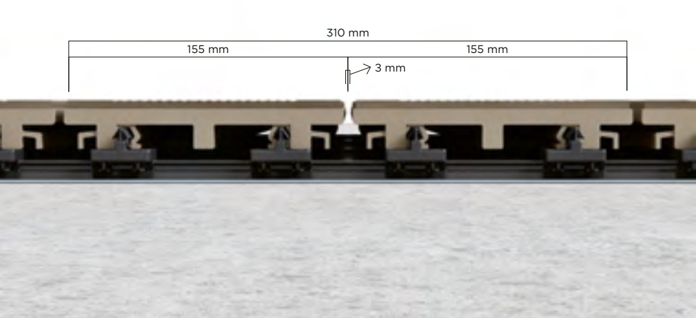
Pormenor da junta (transversal)
